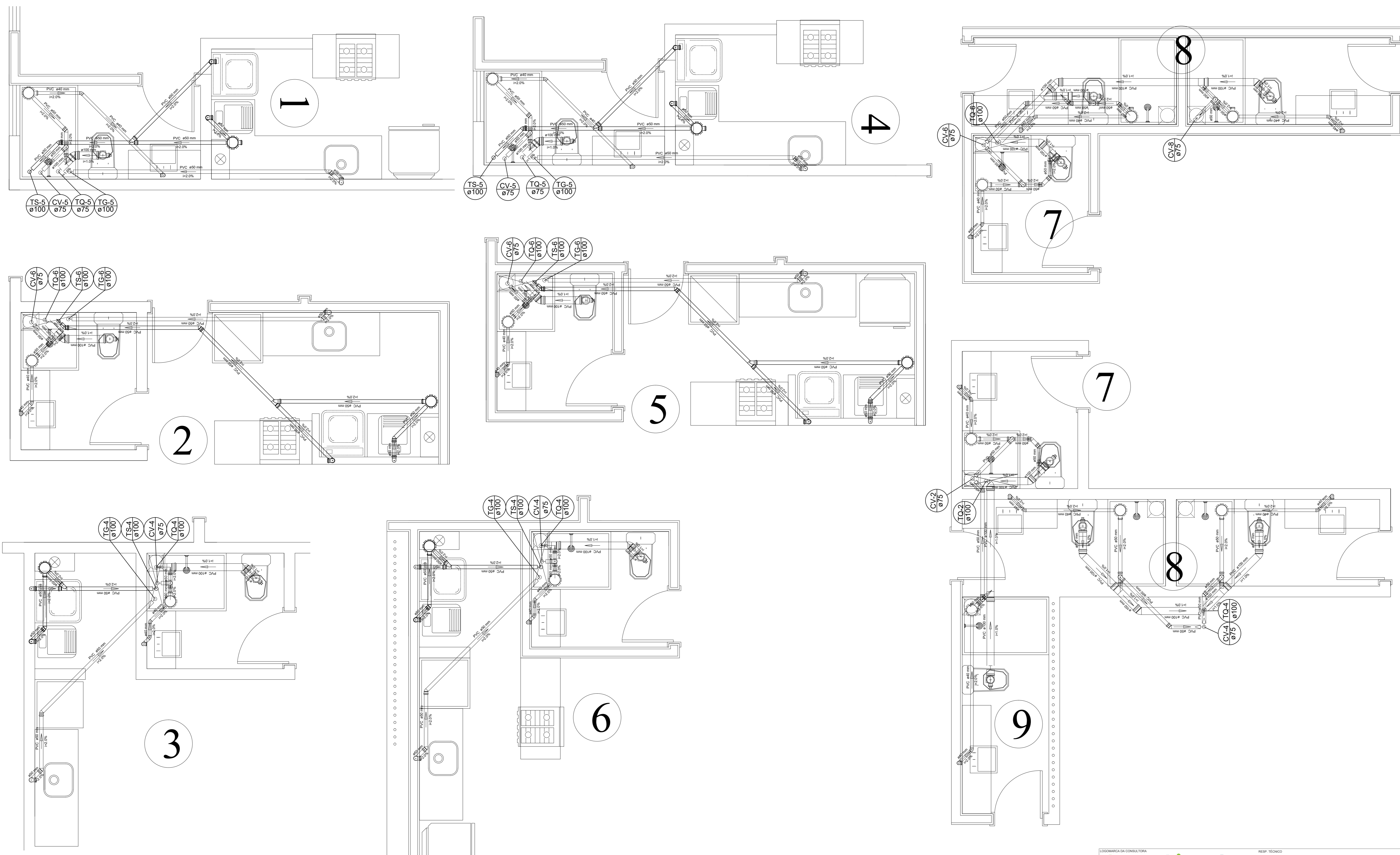
1 DETALHES DE ESGOTO ESCALA 1:25
